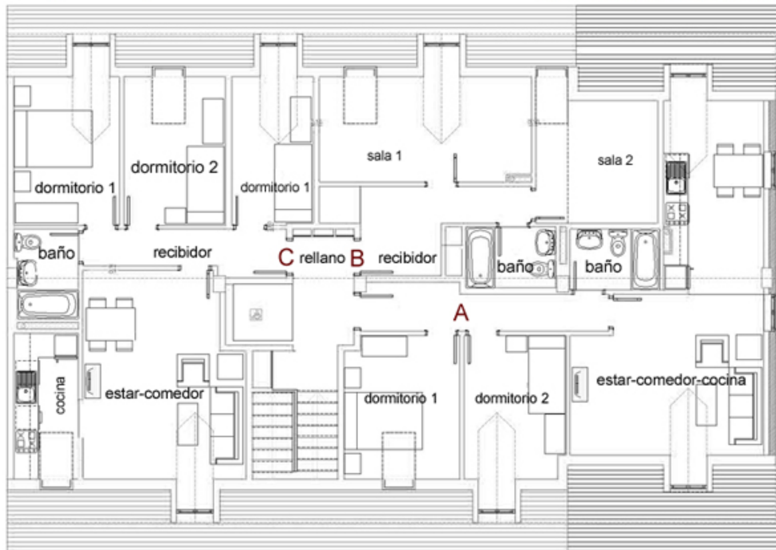
Planta Bajocubierta
